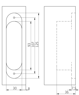
Milling door
