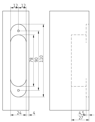
Milling door
