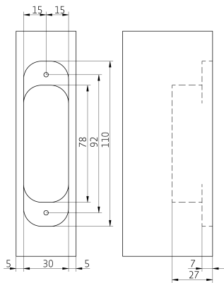
Milling door
