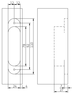
Milling door
