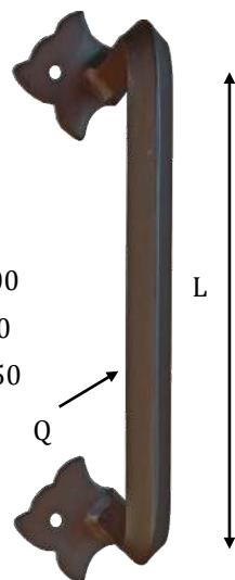
Maniglione zancato Crancked pull handle
