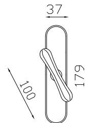
cod. GKA-LLT Cremonese/Martellina con placca Thalassia C.V. Movimento non incluso nel prezzo Cremon/Martellina on Thalassia screw cover plate. Mechanism not included in the price ■ n. 2 pz
