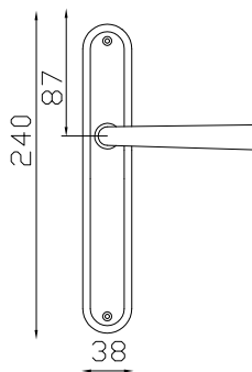
cod. GFR-AAS Maniglia con placca Astra Lever on Astra plate n. 1 set
