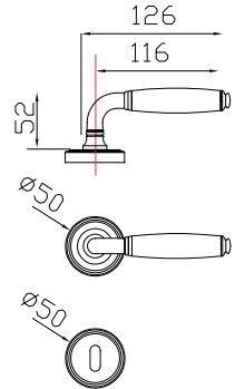
cod. eb. GSB-BAG/pal. GSP-BAG Maniglia con rosetta/bocchetta Gaia Lever on Gaia rose and key hole n. 1 set
