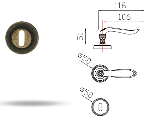
cod. GCR-BAG Maniglia con rosetta/bocchetta Gaia Lever on Gaia rose and key hole ■ n. 1 set
