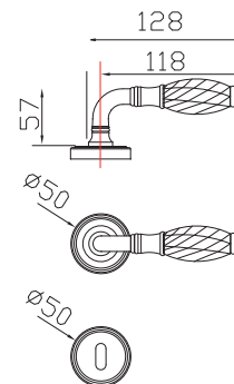
cod. GCW-BAG Maniglia con rosetta/bocchetta Gaia Lever on Gaia rose and key hole ■ n. 1 set
