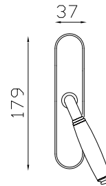
cod. eb. GSB-LMT - cod. pal. GSP-LMT Cremonese/Martellina con placca Thalassia C.V Movimento non incluso nel prezzo Cremon/Martellina on Thalassia C.V screw cover plate Mechanism not included in the price n. 2 pz
