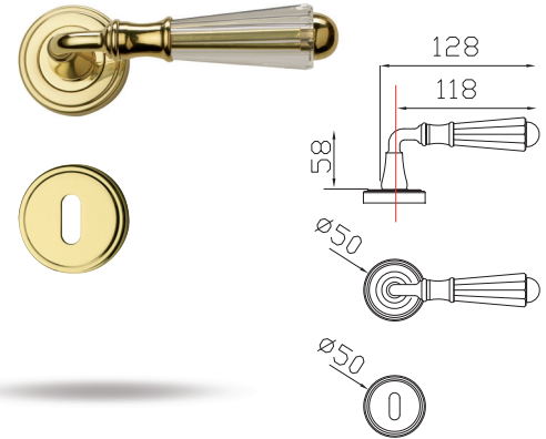
cod. GCX-BAG Maniglia con rosetta/bocchetta Gaia Lever on Gaia rose and key hole n. 1 set
