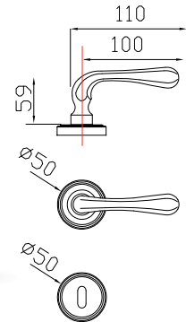
cod. GKA-BAG Maniglia con rosetta/bocchetta Gaia Lever on Gaia rose and key hole ■ n. 1 set
