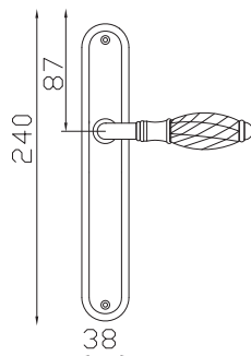
cod. GCW-AAS Maniglia con placca Astra Lever on Astra plate ■ n. 1 set
