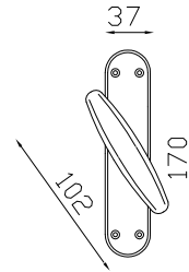
cod. GMX-LA4 (pla)/GMX-LV4 (plb) Cremonese con placca Camilla (634) Cremon on Camilla (634) plate n. 2 pz
