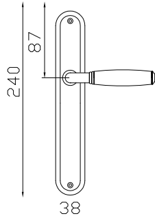
cod. eb. GSB-AAS cod. pal. GSP-AAS Maniglia con placca Astra Lever on Astra plate n. 1 set
