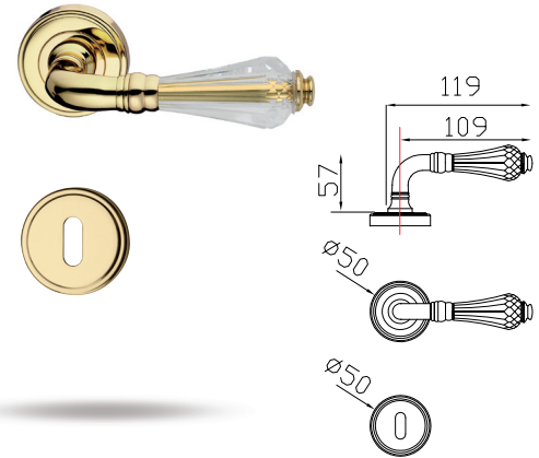
cod. GCY-BAG Maniglia con rosetta/bocchetta Gaia Lever on Gaia rose and key hole ■ n. 1 set
