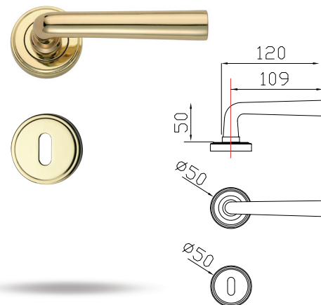
cod. GFR-BAG Maniglia con rosetta/bocchetta Gaia Lever on Gaia rose and key hole n. 1 set
