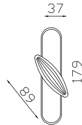
cod. GEL-LLT Cremonese/Martellina con placca Thalassia C.V Movimento non incluso nel prezzo Cremon/Martellina on Thalassia screw cover plate Mechanism not included in the price ■ n. 2 pz
