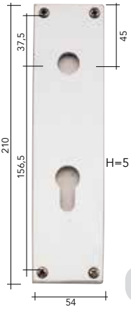
PLACCA PER MANIGLIA / PLATE FOR LEVER HANDLE
