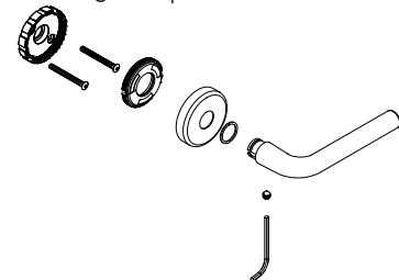
Esempio di applicazione Mounting example
