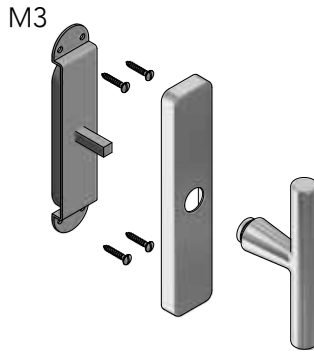
a) Cremonese / Martellina impugnatura a T
