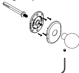
Esempio di applicazione Mounting example
