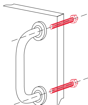
TIPO T SISTEMA DI MONTAGGIO MOUNTING SYSTEM
