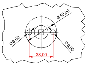
Esempio di applicazione Mounting example
