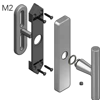
a) Cremonese / Martellina impugnatura a T
