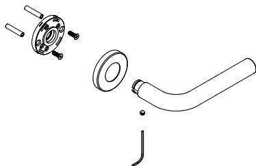
Esempio di applicazione Mounting example
