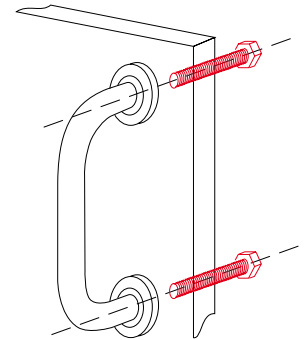
TIPO T SISTEMA DI MONTAGGIO MOUNTING SYSTEM
